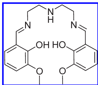
Scheme 1. H 2 valdien Ligand
